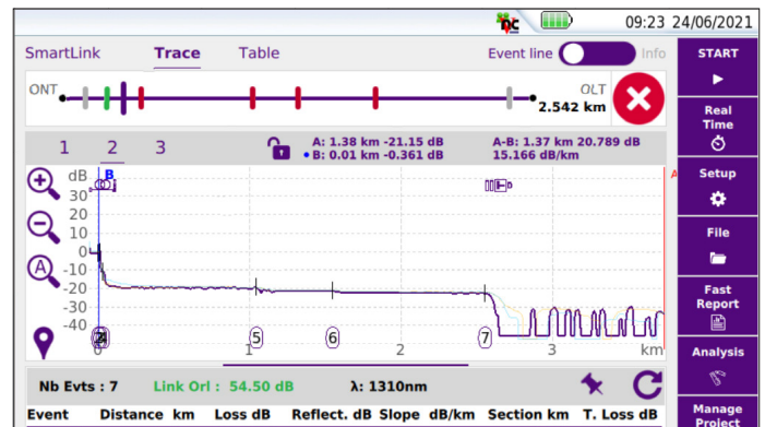
OTDR-Kurvenansicht
